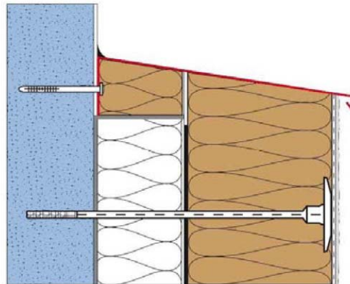
Figure 4e : Profil de couvertine standard + recharge PSE
