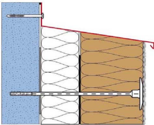
Figure 4d : Profil de départ couvertine inversé
